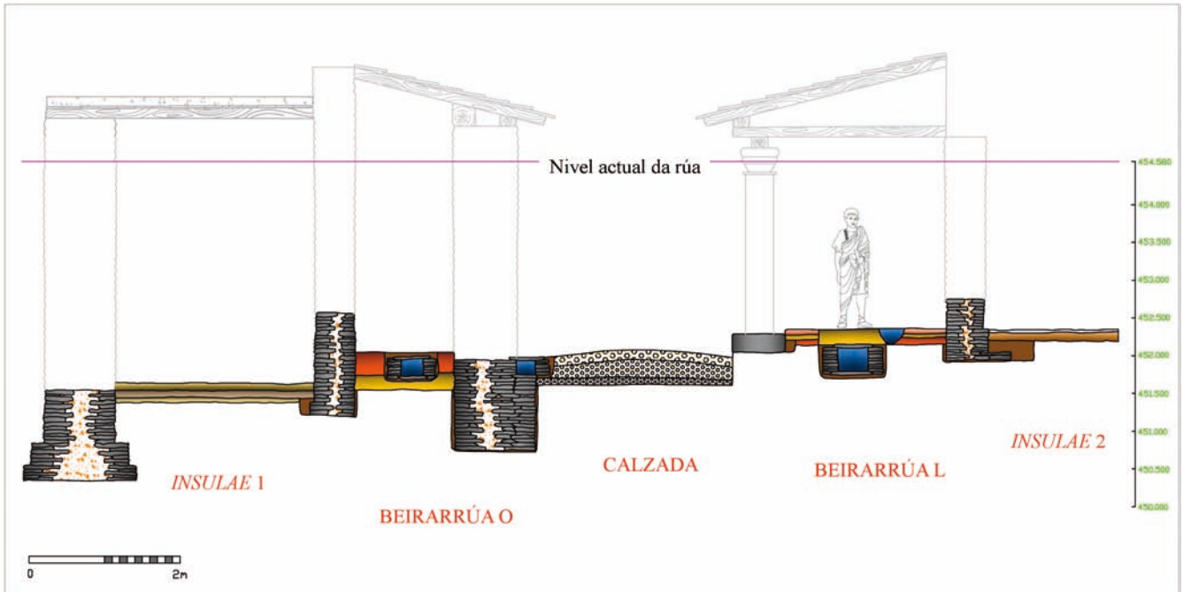
Fig. 25. Reconstrución en sección a través dos restos encontrados.
