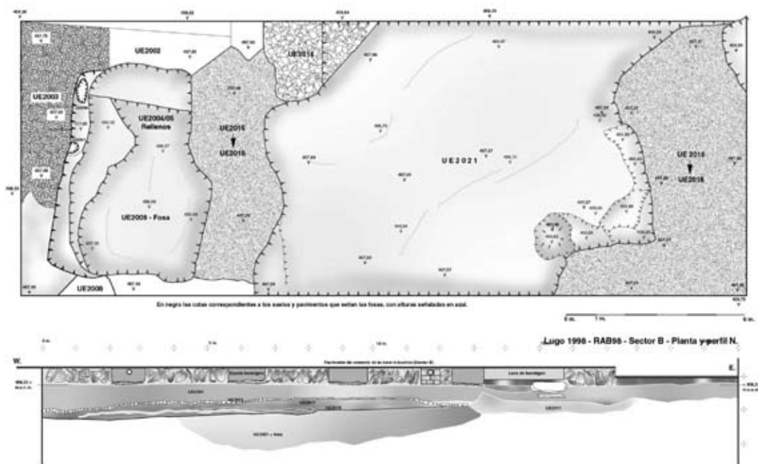
Fig. 31: Planta xeral e perfil norte do sector B
